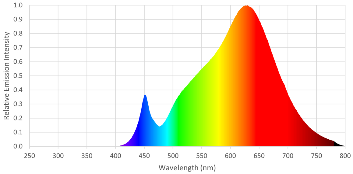
DMS128D27W
